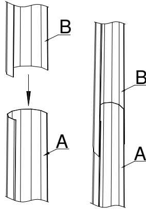
Sıkı geçme Slip joint
